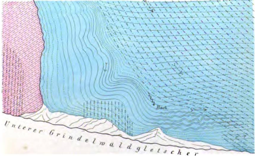
Fig. 8. Gebogene Schieferung im Kalk am Ostfuss des Eiger gegenüber Büregg.
